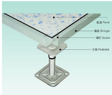
正面 Surface (有边条型 Four PVC edges)
